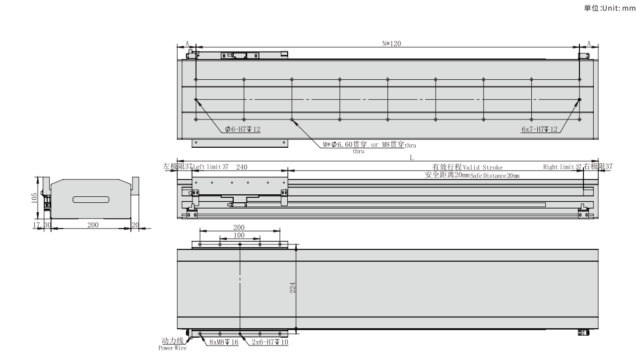
TPA-LNP-200-P22--1023N直线电机 TPA-LNP-200-P22-1023N Linear motor
