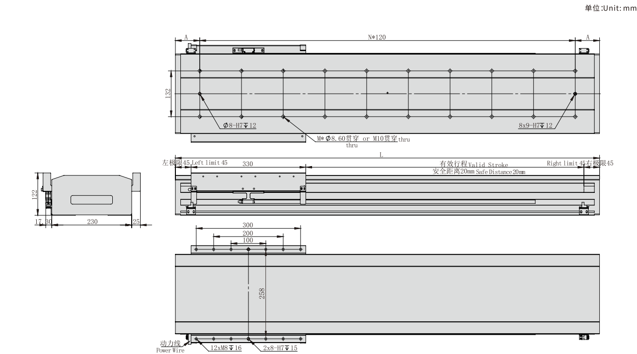
TPA-LNP-230-P33--2469N直线电机 TPA-LNP-230-P33--2469N Linear motor
