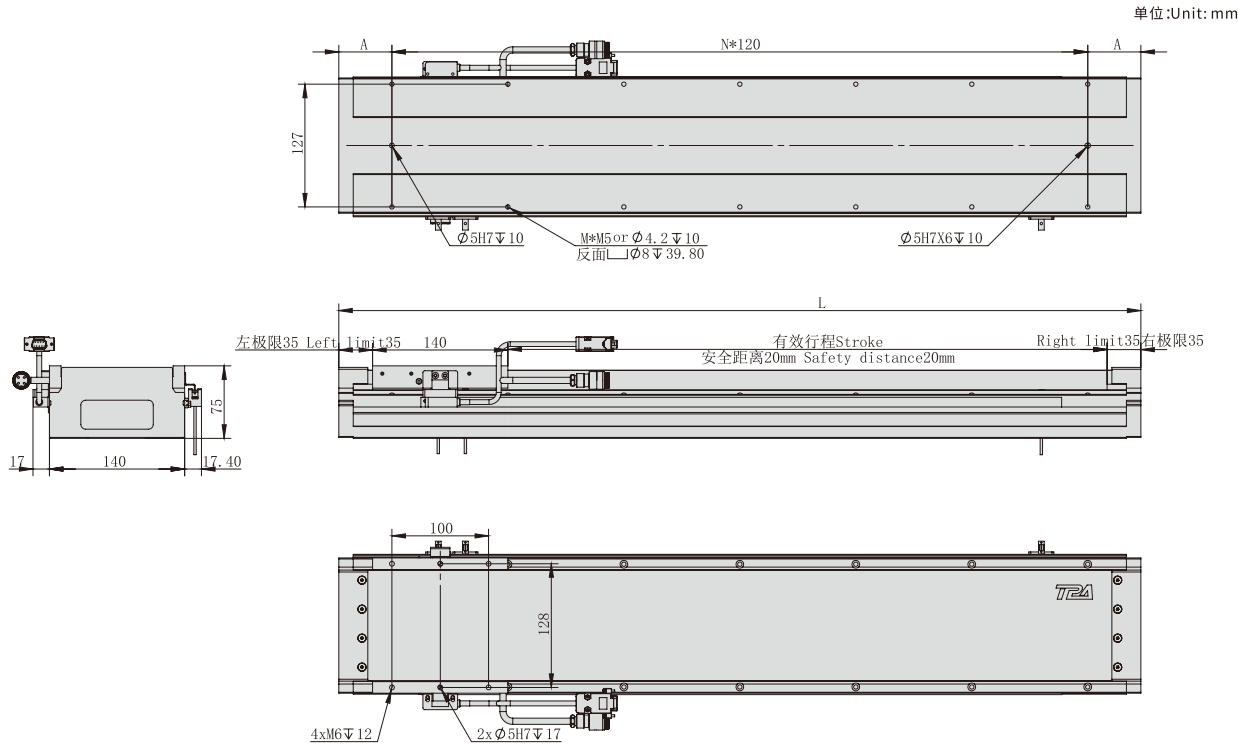
TPA-LNP2-140-20C2--150N直线电机 TPA-LNP2-140-20C2--150N Linear motor
