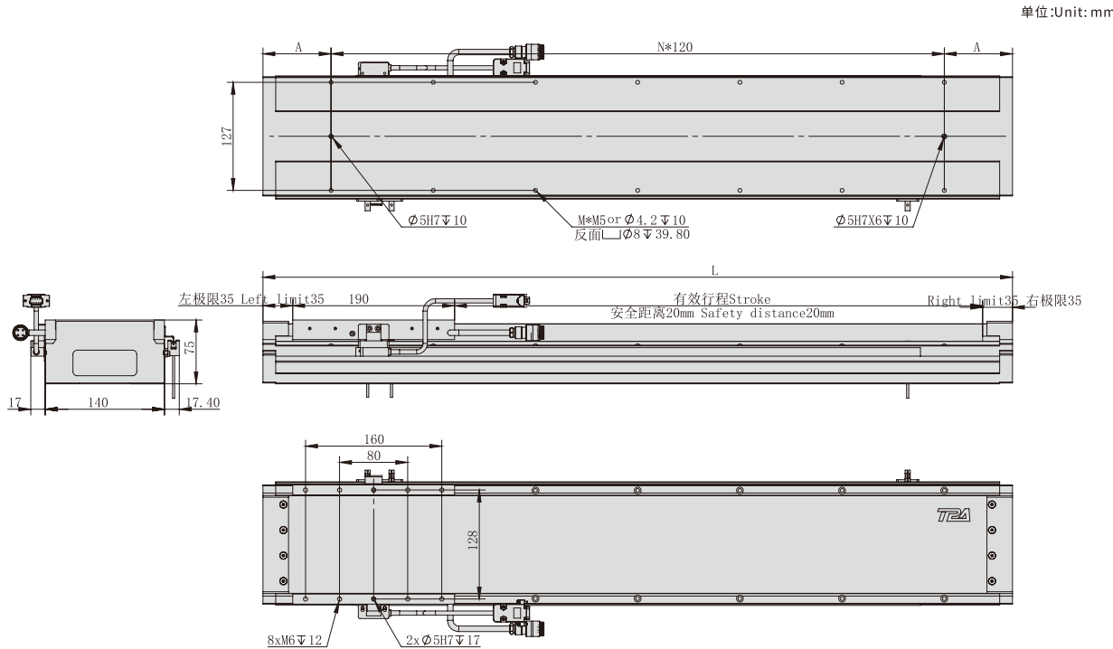
TPA-LNP2-140-20C3--225N直线电机 TPA-LNP2-140-20C3--225N Linear motor
