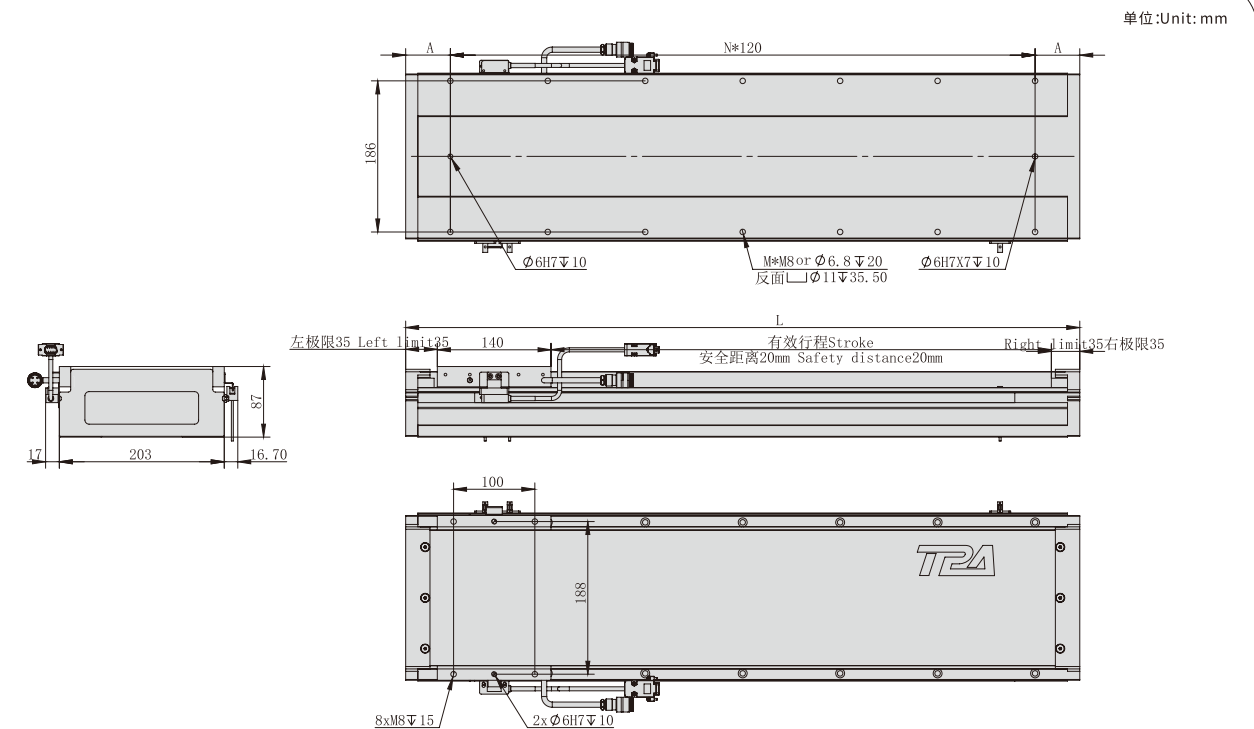
TPA-LNP2-200-55C2--418N直线电机 TPA-LNP2-200-55C2--418N Linear motor
