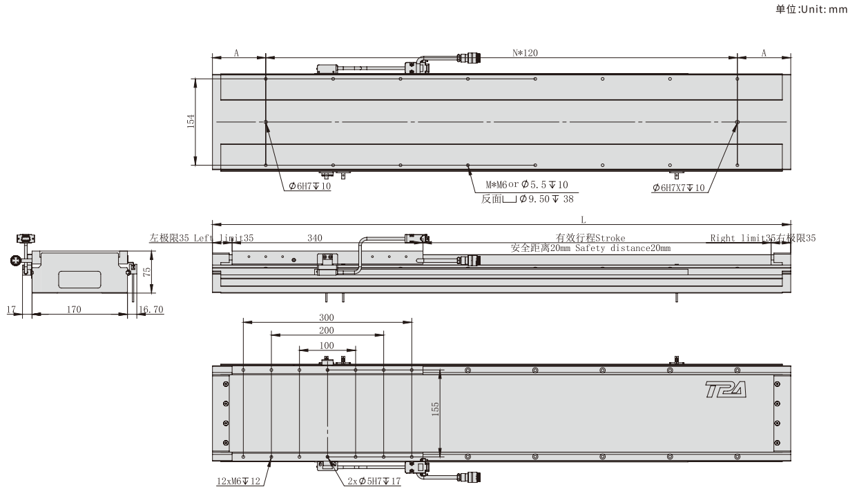
TPA-LNP2-170-35C6--798N直线电机 TPA-LNP2-170-35C6--798N Linear motor
