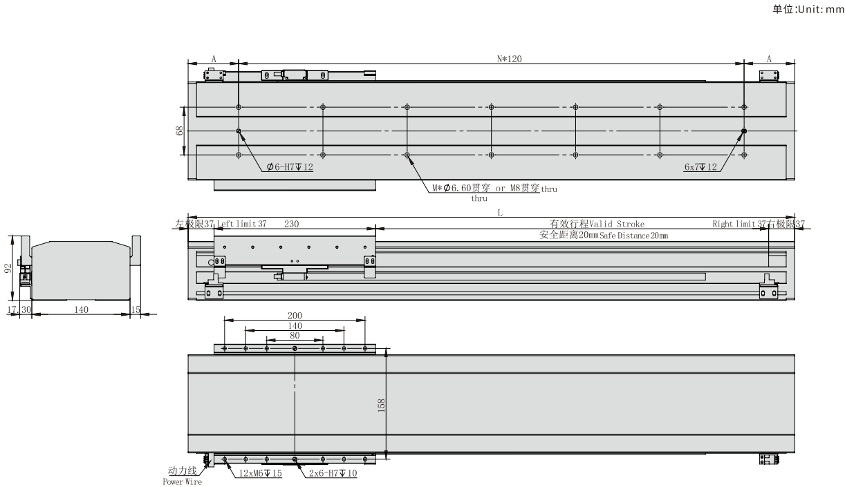
TPA-LNP-140-P12--579N直线电机 TPA-LNP-140-P12--579N Linear motor
