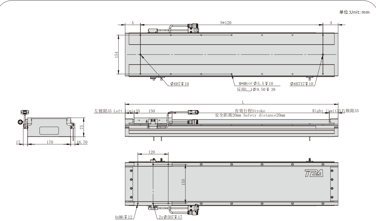
TPA-LNP2-170-35C2--265N直线电机 TPA-LNP2-170-35C2--265N Linear motor
