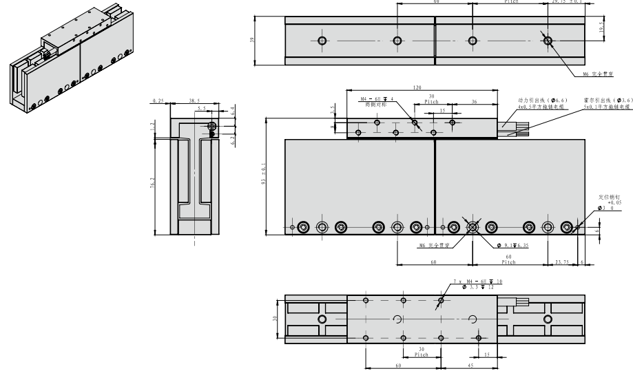
TPA动 定子尺寸图 TPA Dimension diagram of Mover & stator
