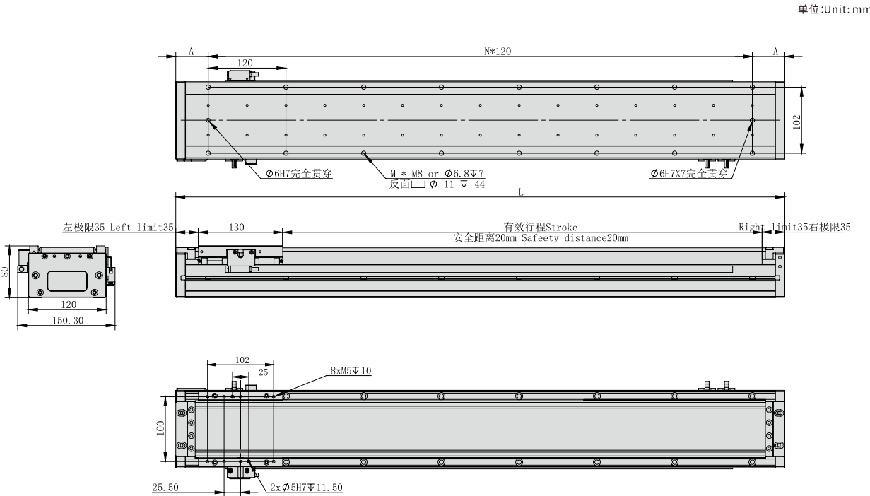
TPA-LNP3-120-35C2--265N直线电机 TPA-LNP3-120-35C2--265N Linear motor
