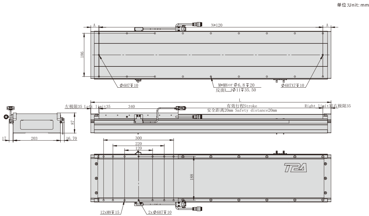
TPA-LNP2-200-55C6--1253N直线电机 TPA-LNP2-200-55C6--1253N Linear motor
