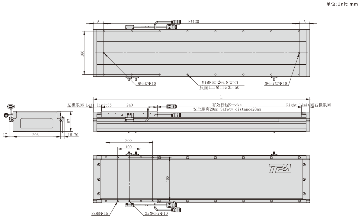
TPA-LNP2-200-55C4--835N直线电机 TPA-LNP2-200-55C4--835N Linear motor
