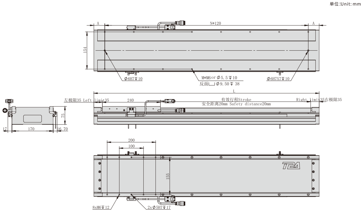
TPA-LNP2-170-35C4--532N直线电机 TPA-LNP2-170-35C4--532N Linear motor
