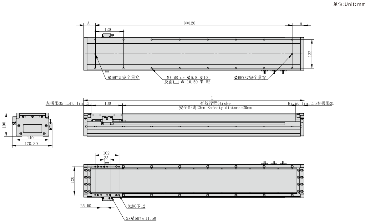
TPA-LNP3-140-55C2--418N直线电机 TPA-LNP3-140-55C2--418N Linear motor
