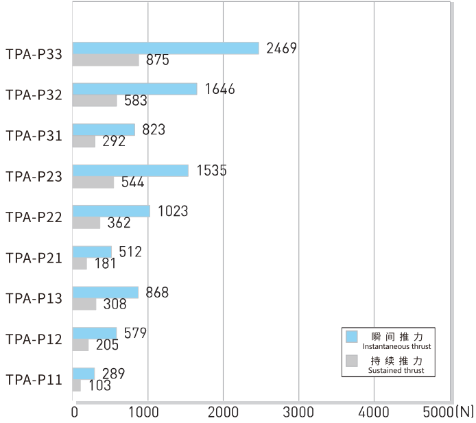
马达推力图 Motor thrust diagram
