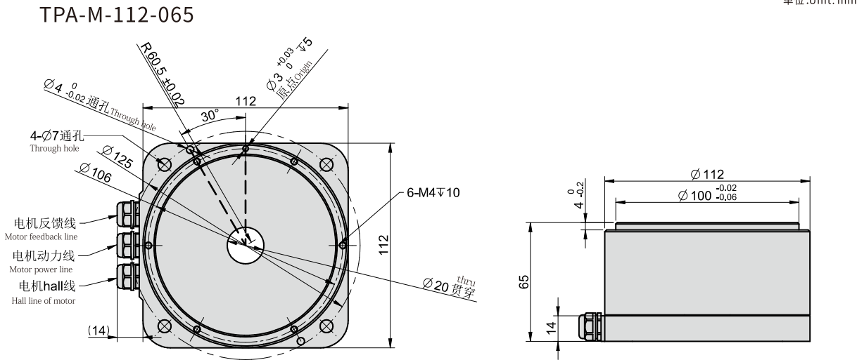
安装尺寸图 Installation dimension drawing
