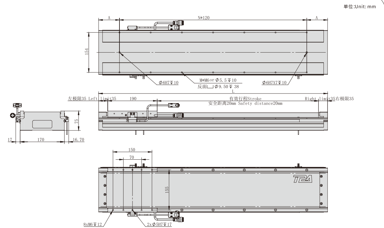
TPA-LNP2-170-35C3--395N直线电机 TPA-LNP2-170-35C3--395N Linear motor
