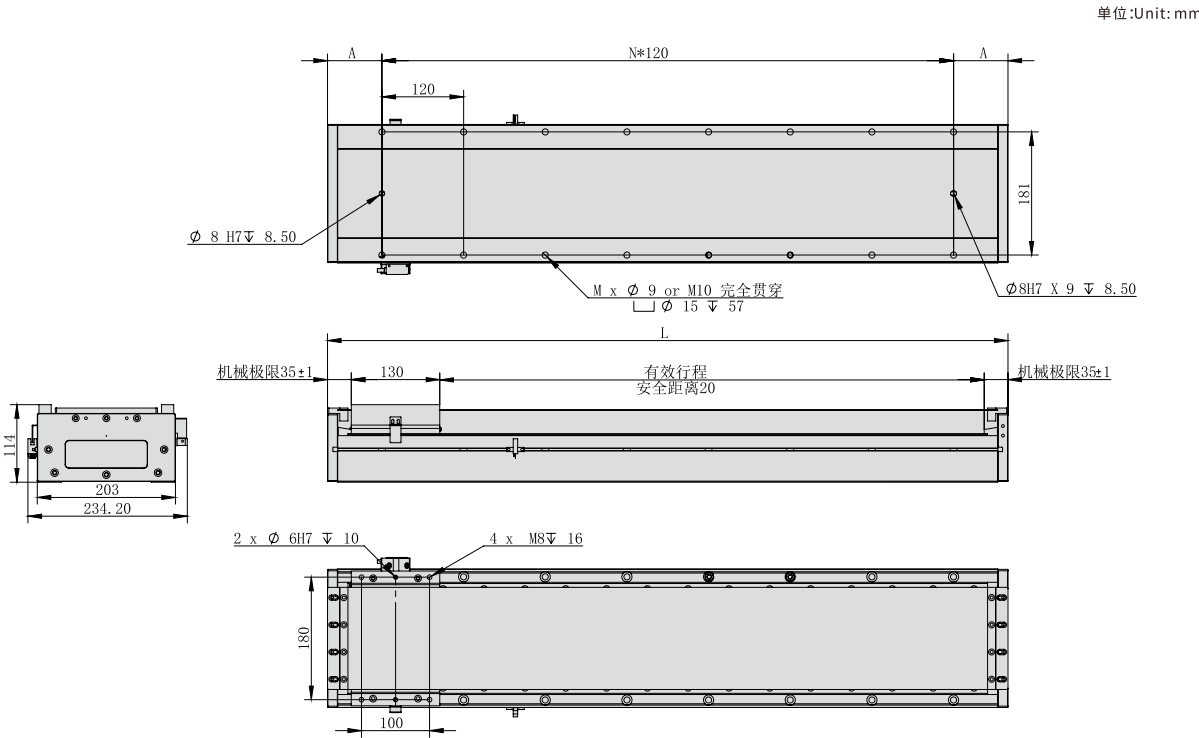
TPA-LNP3-200-100C2-759N直线电机 TPA-LNP3-200-100C2--759N Linear motor
