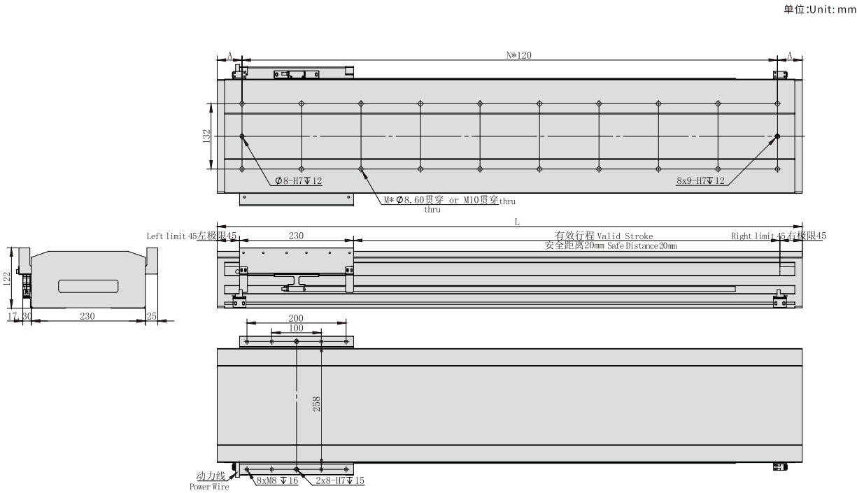
TPA-LNP-230-P32--1646N直线电机 TPA-LNP-230-P32--1646N Linear motor
