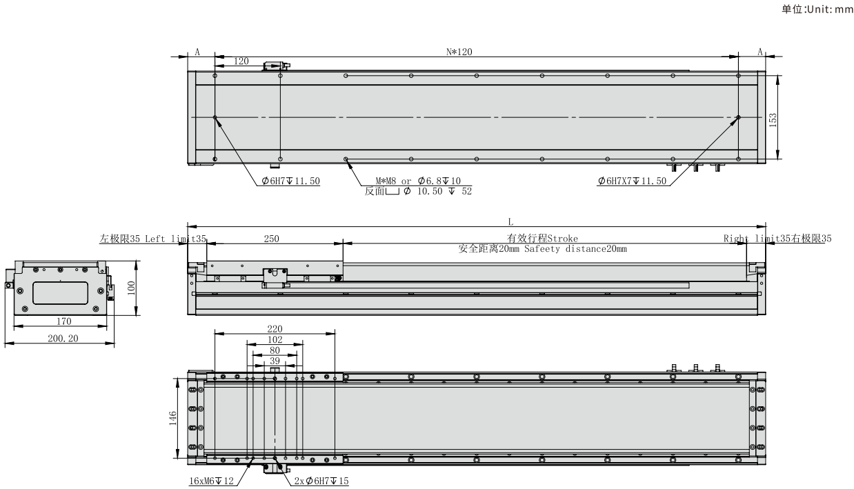
TPA-LNP3-170-75C4-1132N直线电机 TPA-LNP3-170-75C4--1132N Linear motor
