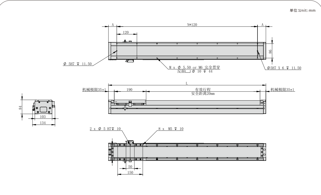
TPA-LNP3-100-20C3--225N直线电机 TPA-LNP3-100-20C3--225N Linear motor
