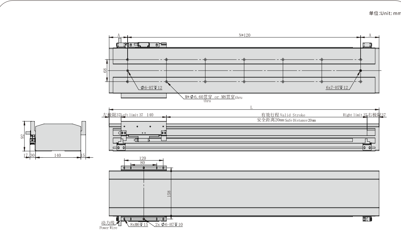
TPA-LNP-140-P11--289N直线电机 TPA-LNP-140-P11--289N Linear motor
